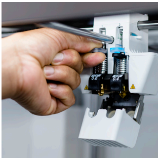
Print core CC 0,6 mm Muni d'un rubis pour l'impression de composites abrasifs de fibres de carbone et de verre
