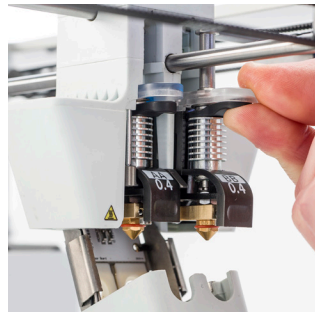
Print core AA et BB 0,25, 0,4, 0,8 mm Buses rapidement interchangeables pour matériau de construction et supports solubles
