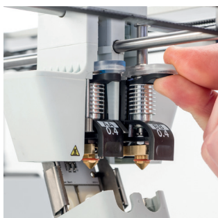
Print core AA 0,25, 0,4, 0,8 mm Le changement rapide minimise les temps d'arrêt
