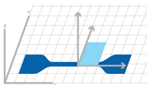
Dim.(mm) : 75x1 2,5x2 Eprouvette de type ISO 527-5A
